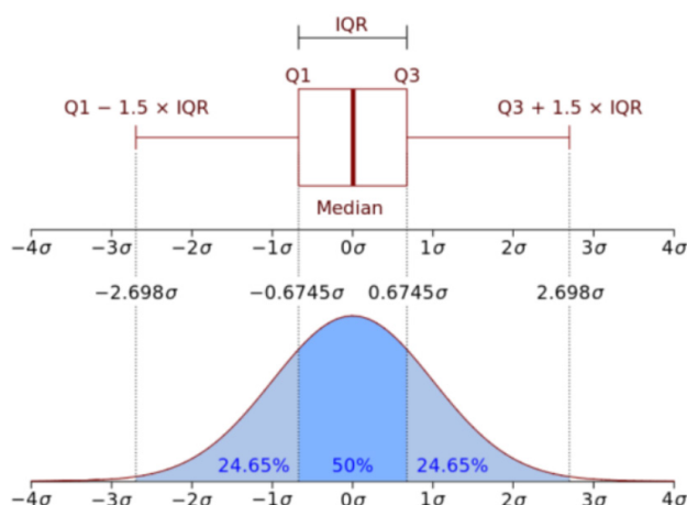
Рис. 7. Пример распределения выбросов в базе данных.
